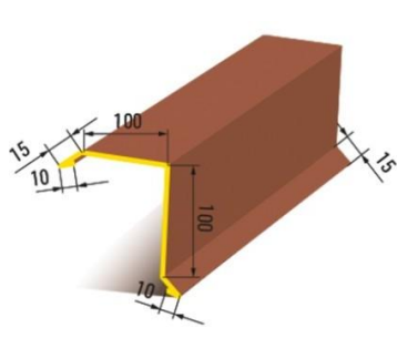
Závětrná lišta horní
